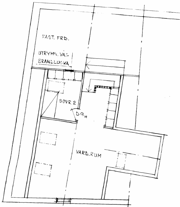
VINDSPLAN 1:100 (LÄGENHET 1.)
