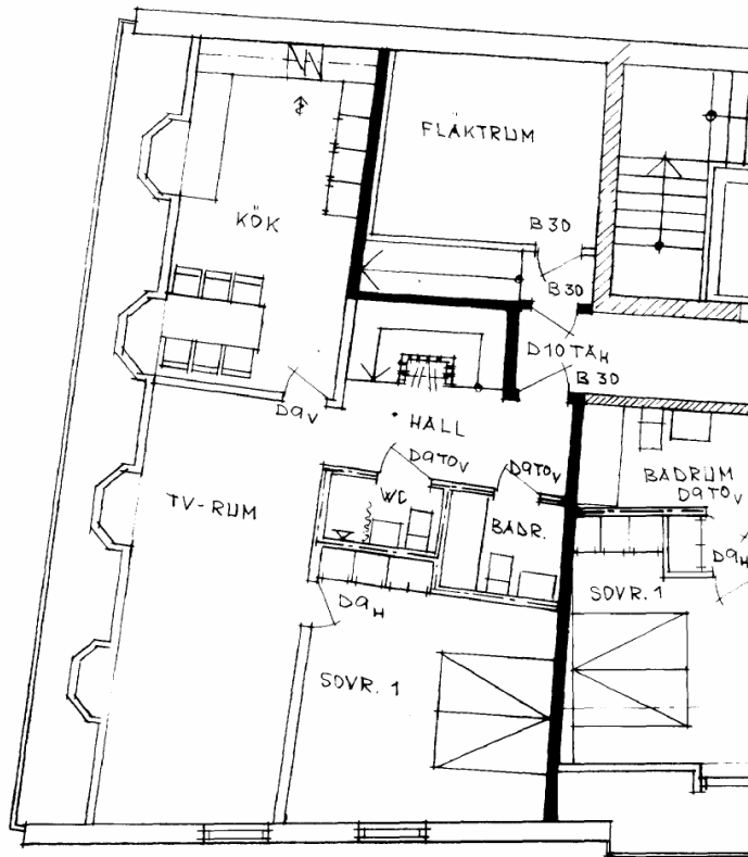
PLAN 4 1:100
